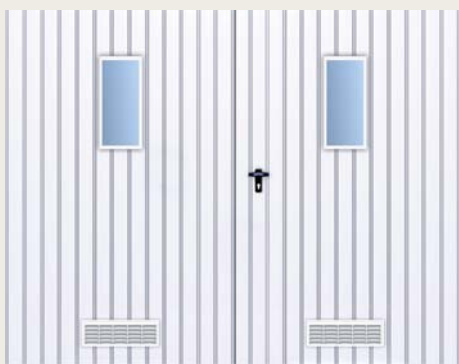
Brama rozwierna dwuskrzydłowa wypełniona blachą T-10, układ wypełnienia pionowy, brama z okienkami w układzie pionowym oraz z kratką wentylacyjną
