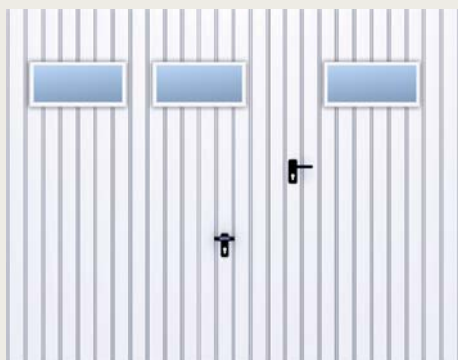
Brama z drzwiami przejściowymi wypełniona blachą trapezową T-10, układ wypełnienia pionowy, brama oraz drzwi przejściowe z okienkami w układzie poziomym
